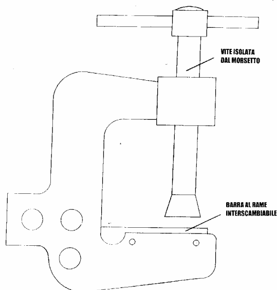
APERTURA MORSETTO: MM. 90
